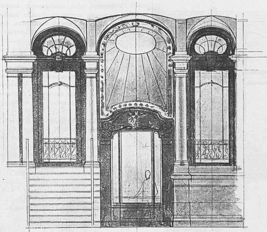
491. Вариантъ обработки вестибюля (поперечный разрѣзь).
